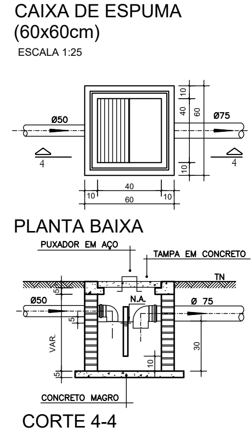
PLANTA BAIXA CORTE 4-4
