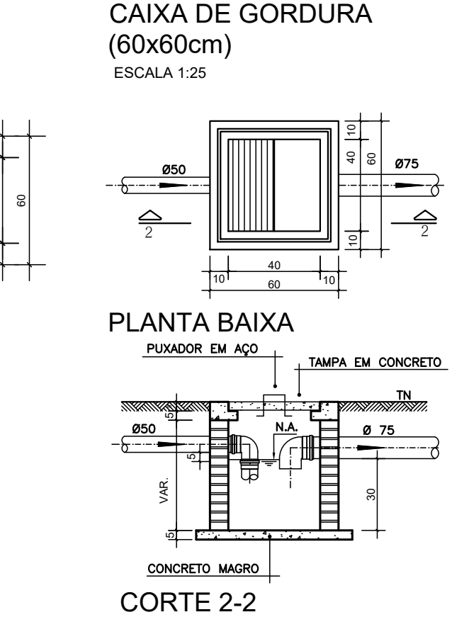
PLANTA BAIXA CORTE 2-2
