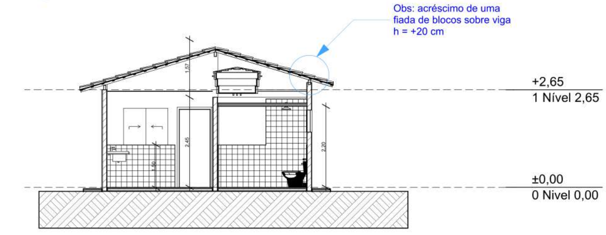
Corte 1:100
