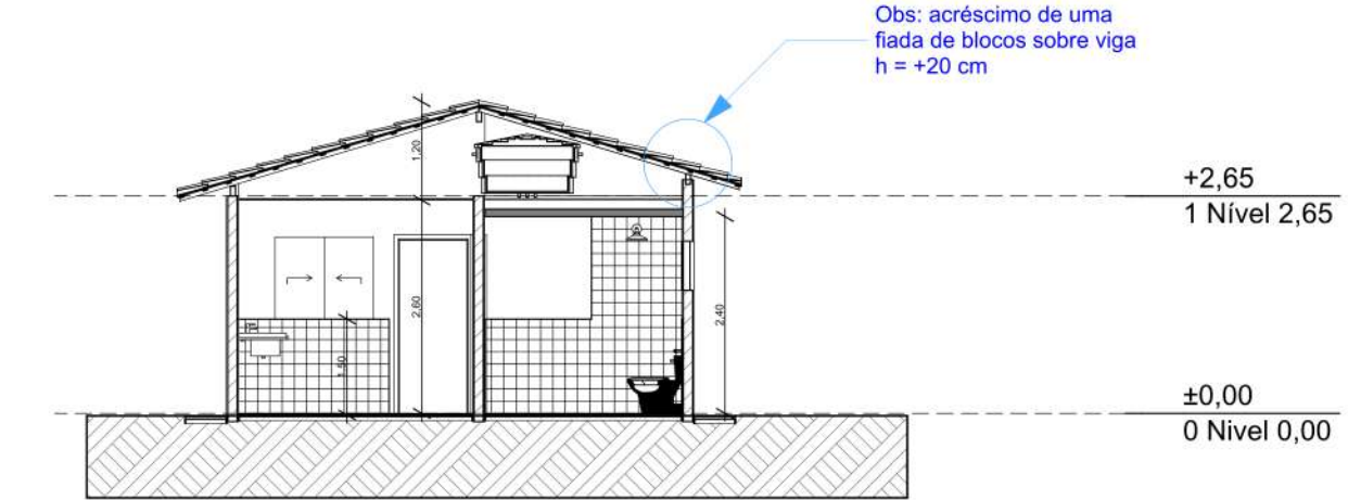
Corte 1:100
